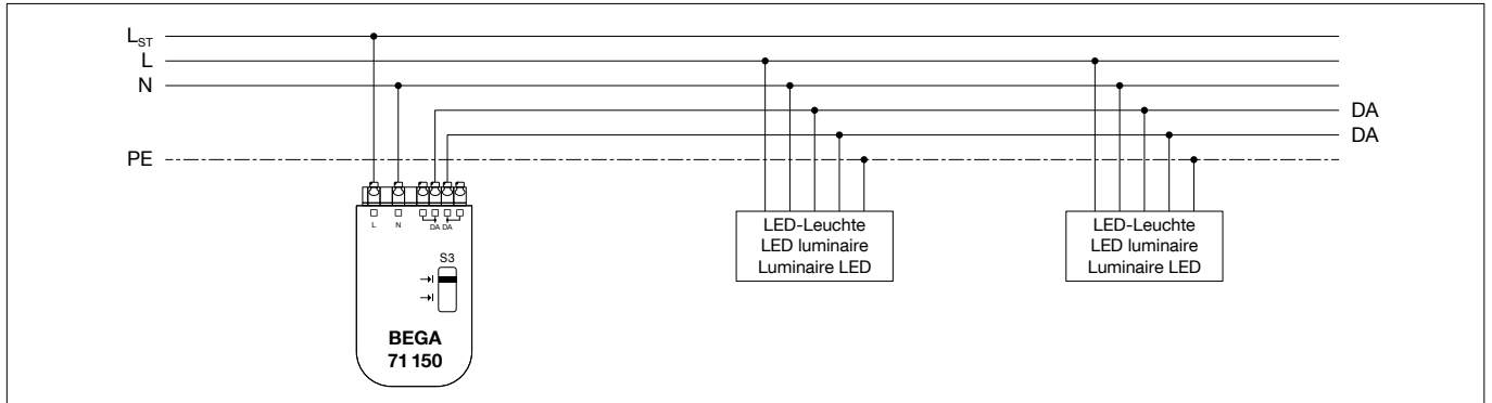
Schaltbild Betriebsart 1
