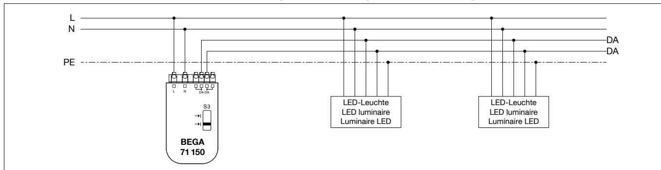
Schaltbild Betriebsart 2
